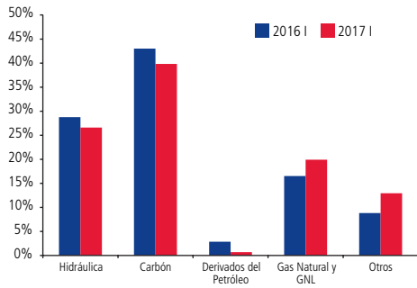
GRÁFICO 8 Composición de la generación eléctrica por tipo de combustible
