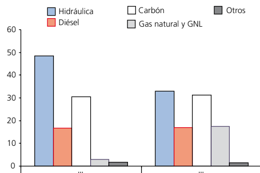
Composición de la generación eléctrica por tipo de combustible (porcentaje)
