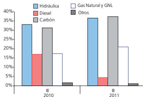
Composición de la generación eléctrica por tipo de combustible
