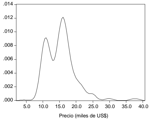
Estados Unidos Kernel Density (Normal, h = 11.682 )
