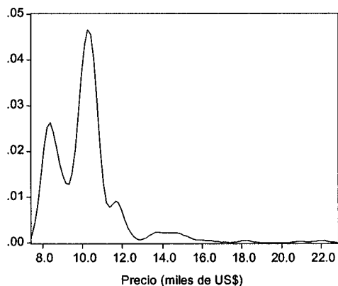
Estados Unidos Kernel Density (Normal, h = 3.1488 )
